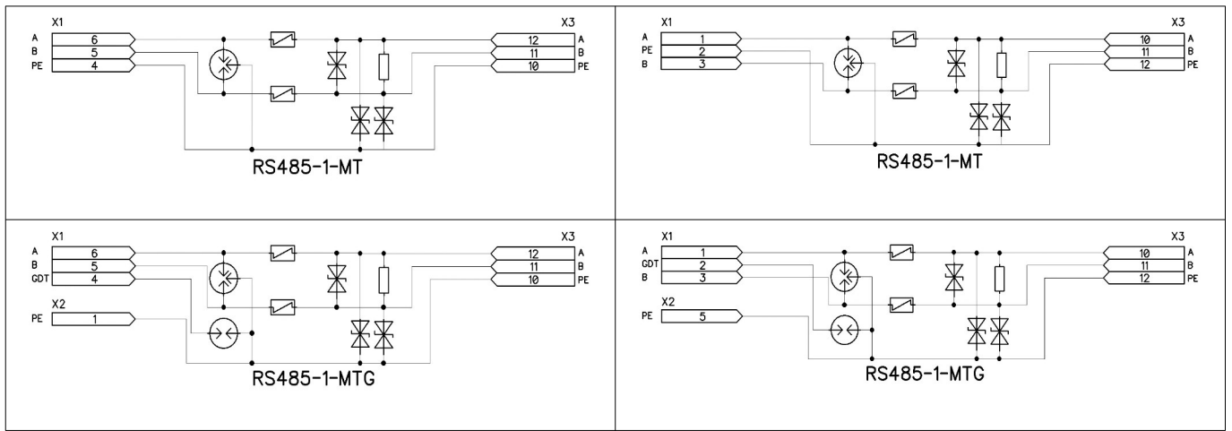
Рис. 1. Принципиальные схемы Исполнение 1 слева Исполнение 2 справа
