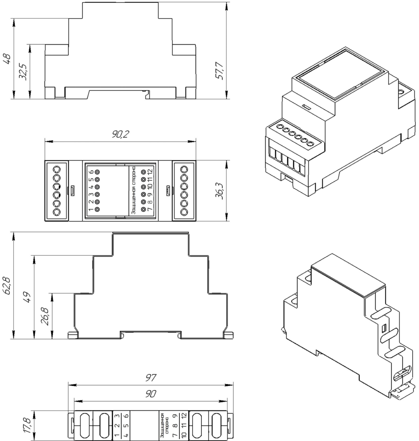
Рис. 2. Установочные размеры Исполнение 1 сверху Исполнение 2 снизу
