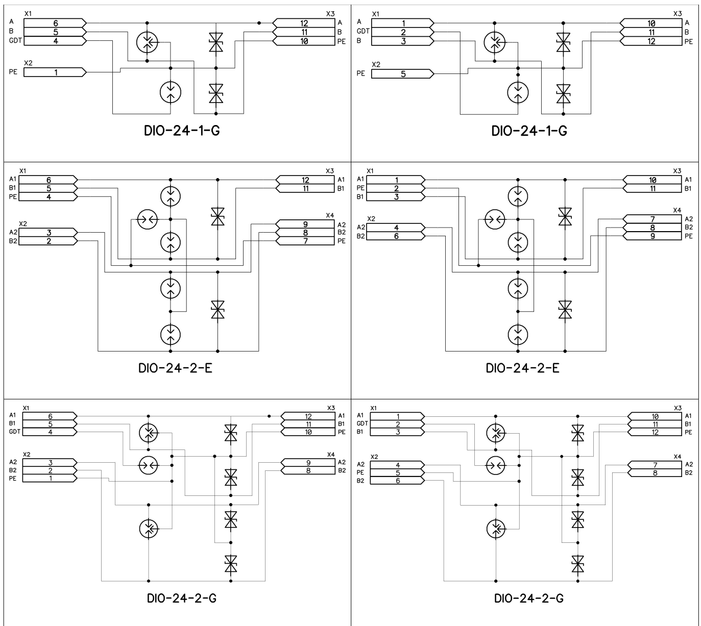
Рис. 1. Принципиальные схемы Исполнение 1 слева Исполнение 2 справа
